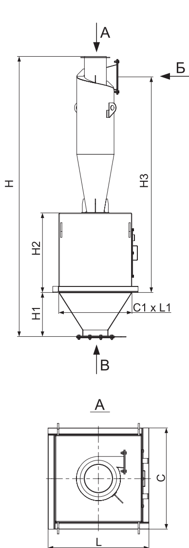
ЦН-15-1П
