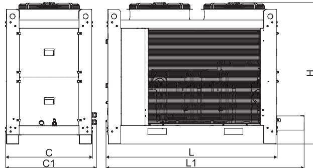
BasicAir/UnicAir-C-40...C-65
